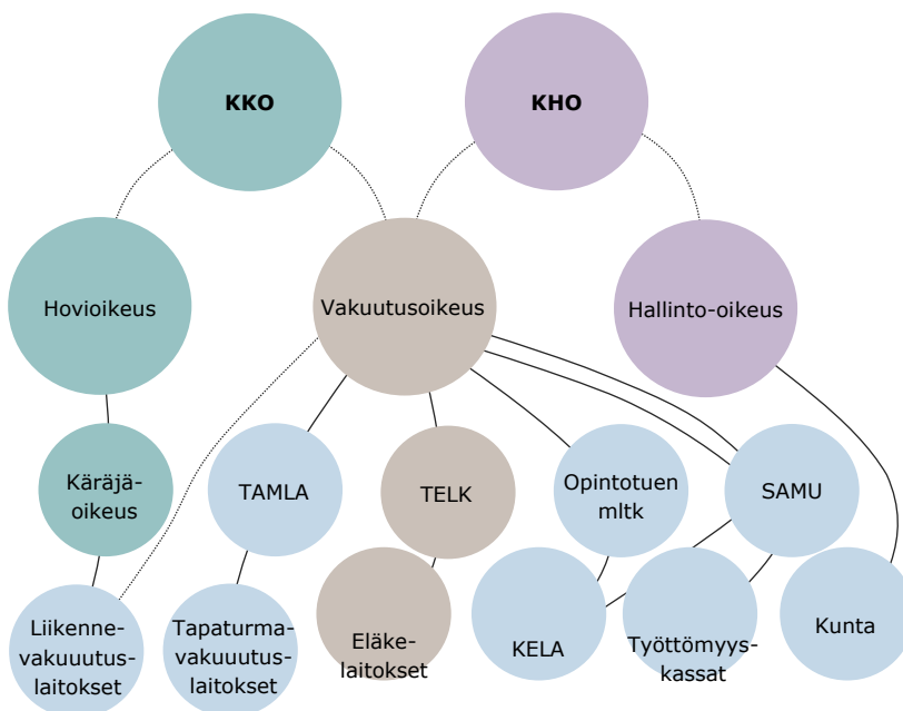
Kuva 1. Sosiaalivakuutuksen muutoksenhakujärjestelmä
